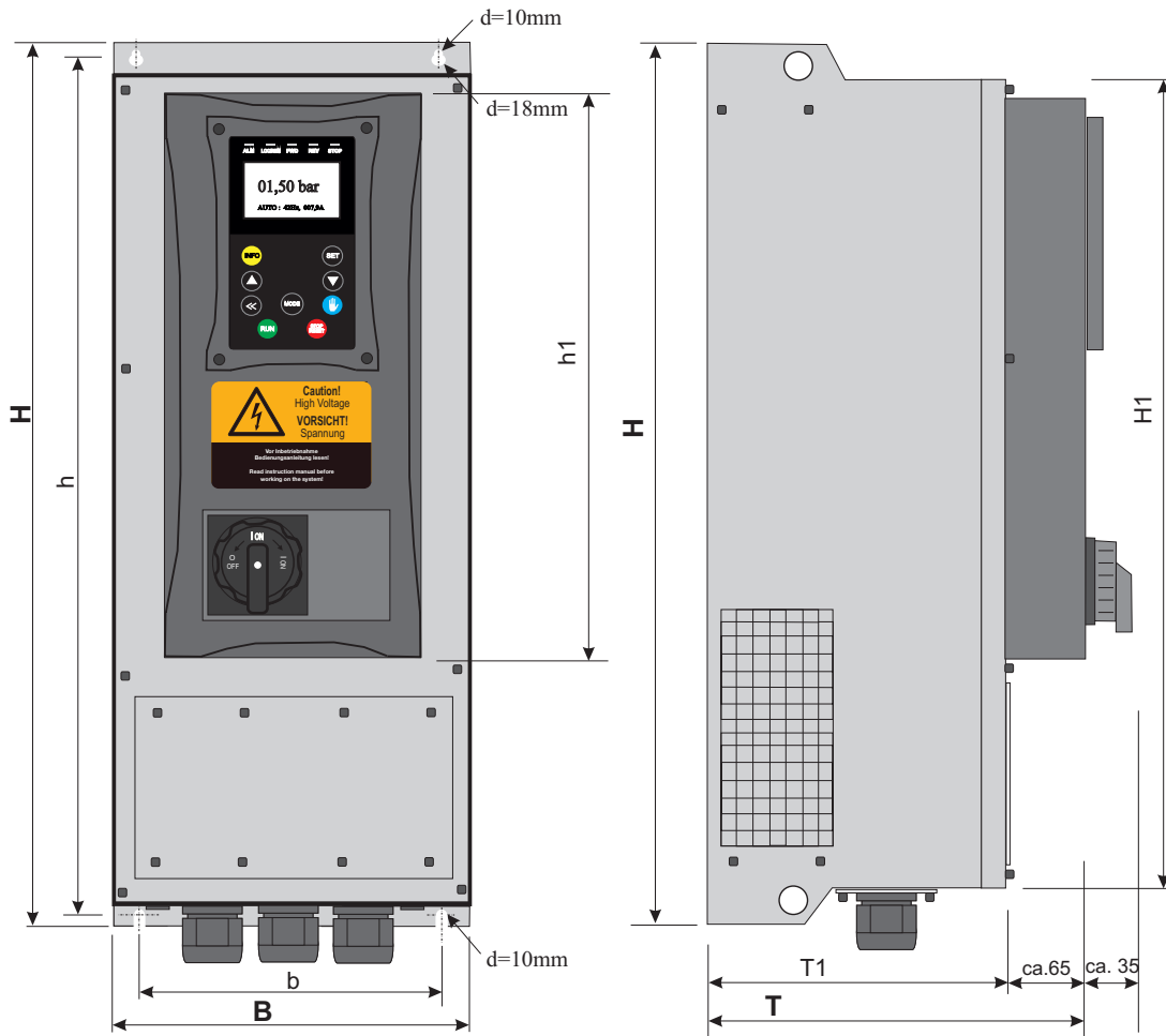
Einzelregler mit Reparaturschalter, MARE Regler Version 2 Größe 3 + 4,
